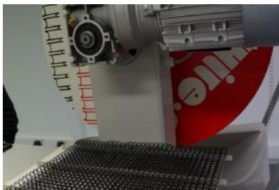
Podávání cívek i formátovaných hřbetů twin-wire.
